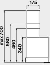
Vista laterale con camino opzionale
