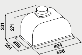
Foro per incasso 50 cm: 262 x 506 mm
