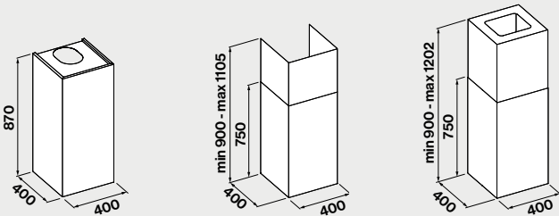
Parete Parete telescopica Isola
