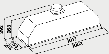
105 cm: 262 x 1029 mm
