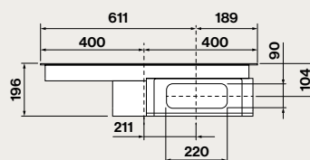
Vista posteriore
