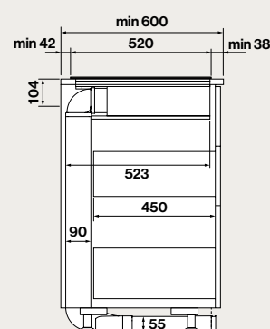
Vista laterale con KACL.1071
