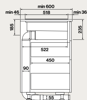
Vista laterale con KACL.1071
