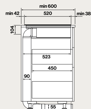
Vista laterale con KACL.1071
