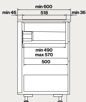
Vista laterale con tubo telescopico in dotazione
