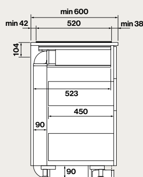
Vista laterale con KACL.1075
