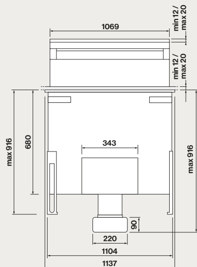
Vista frontale
