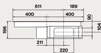
Vista posteriore
