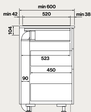
Vista laterale con KACL.1072
