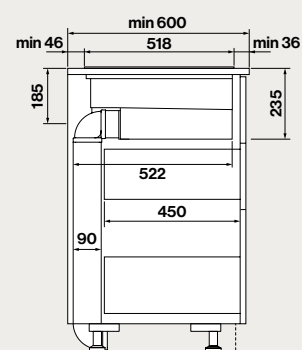
Vista laterale con KACL.1072
