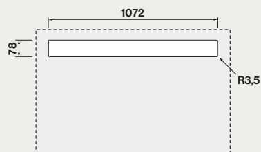
Dimensioni foro
