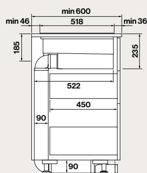
Vista laterale con KACL.1075
