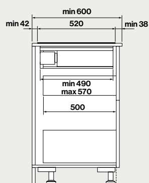
Vista laterale con tubo telescopico in dotazione
