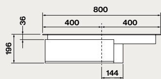
Vista frontale
