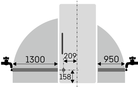
IceMaker con allacciamento fisso alla rete idrica - attacco 3/4 " Il tubo flessibile di 3 m è disponibile come accessorio
