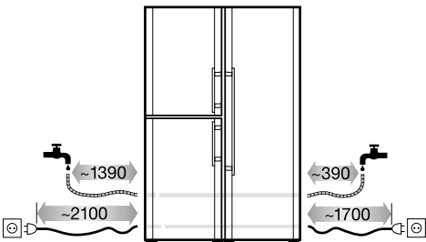
IceMaker con allacciamento fisso alla rete idrica - attacco 3/4 " Il tubo flessibile di 3 m è disponibile come accessorio
